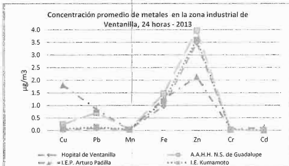
Gráfico N° 3. La concentración promedio de metales en el aire (durante 4 días) muestra concentraciones altas de Zinc en las 4 estaciones de monitoreo, seguidas por Hierro y Cobre. Dichos resultados no exceden los valores referenciales de 24 horas, del Criterio de Calidad de Aire Ambiental (AAQC) de Canadá. Sin embargo, sobrepasa los valores referenciales para plomo y cadmio, de 0,5 y 0,025, respectivamente. Fuente: DIRESA-Callao.
