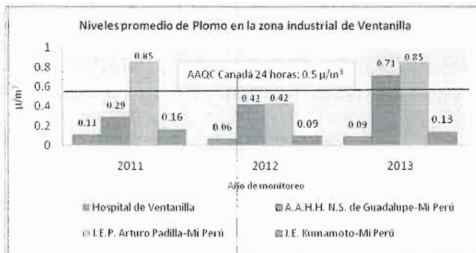
Gráfico N° 1. El nivel promedio diario de Plomo en la estación de I.E.P. Arturo Padilla superan los niveles estándar referenciales de AAQC-Ambient Air Quality Criterion, o Criterio de Calidad de Aire Ambiental (AAQC) de Canadá para 24 horas, los años 2011 y 2013. Se observa la misma situación en la estación el AA.HH. Nuestra Señora de Guadalupe en el año 2013. Fuente: Informe N° 33-2012-GRS/GRS/DESA/DEPAYSO/EPA/VCAR, de Diresa-Callao.
