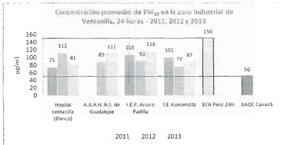
Gráfico N° 2. La concentración de PM_{10} (partículas menores a 10 micras), 24 horas, no sobrepasan el ECA los tres años y en todas las estaciones, sin embargo, si sobrepasa el AAQC Canadá en todos los puntos de monitoreo y años. Fuente: DIRESA-Callao.
